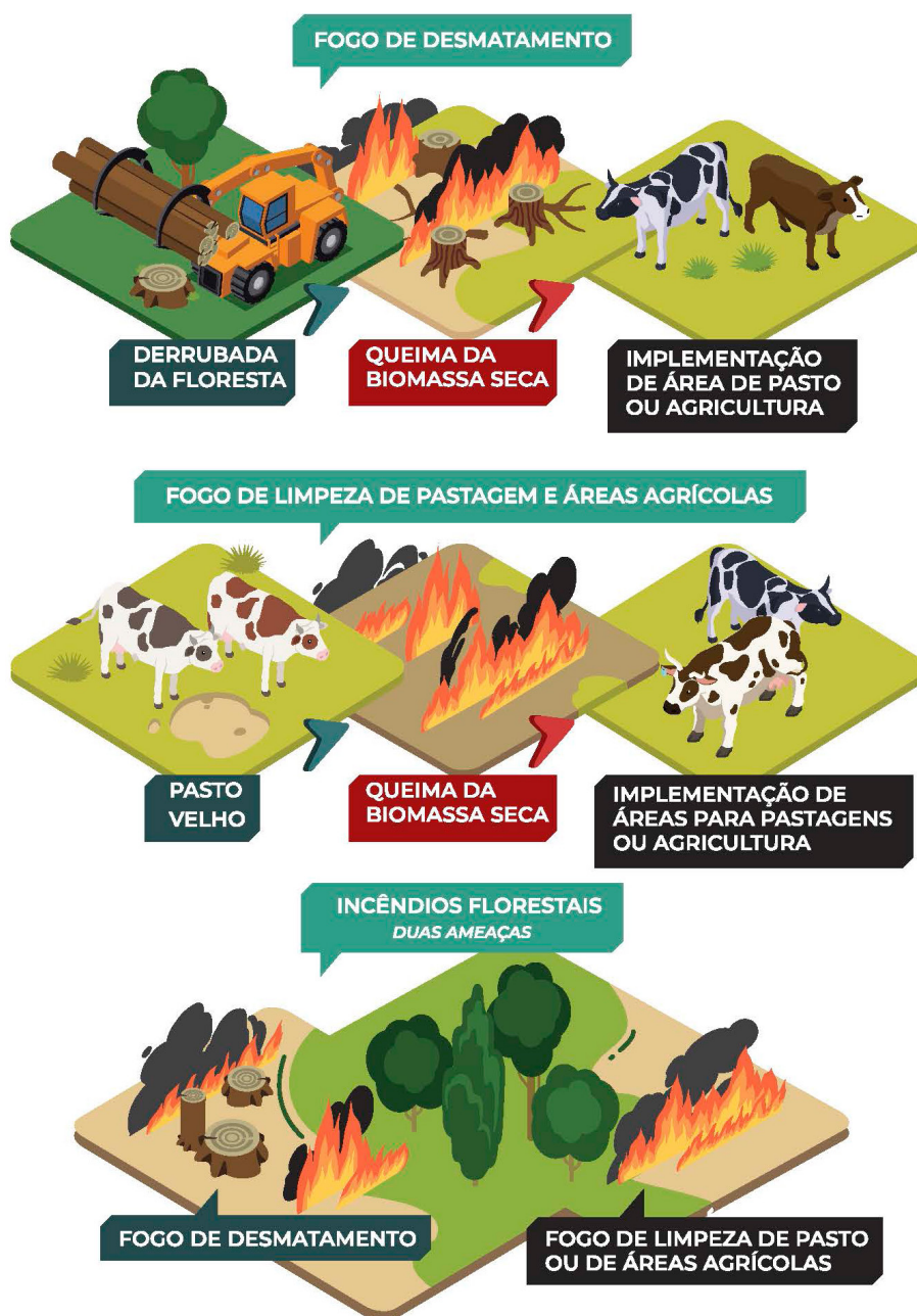
Figura 2. Desenho esquemático sobre os tipos de fogo comumente utilizados na Amazônia. Fonte: IPAM, 2020.
